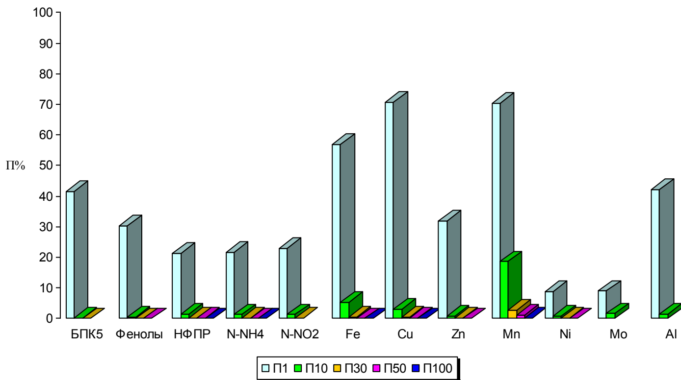
Рис. 3 Соотношение повторяемостей (II) концентраций разного уровня отдельных загрязняющих веществ в поверхностных водах Российской Федерации в 2014 г.
