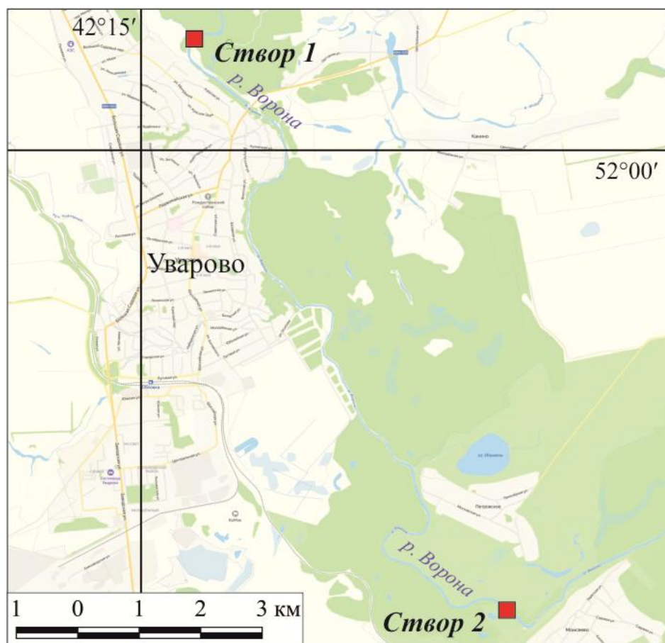
Рисунок 1 – Карта-схема расположения гидрохимических створов
