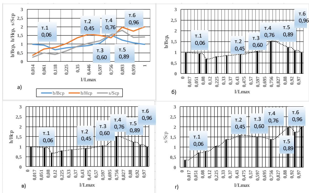
Рисунок 1– Нормированные морфометрические характеристики Таганрогского залива: комплексный график b/B_{\text{ср.}} , h/H_{\text{ср.}} , s/S_{\text{ср.}} (а), нормированной: ширины (б), глубины (в), площади поперечного сечения (г)
