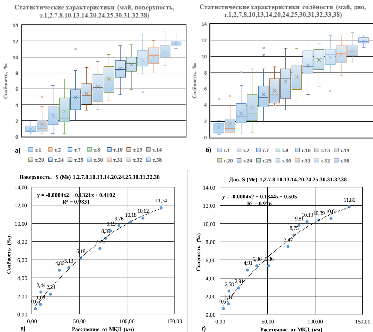
Рисунок 3 – Статистические характеристики солёности (т.1,2,7,8,10,13,14,20,24,25,30,31,32,33,38): поверхность (а), дно (б).
