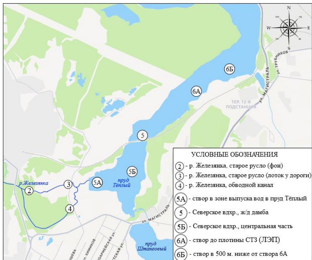
Рисунок 1 – Расположение створов исследования
